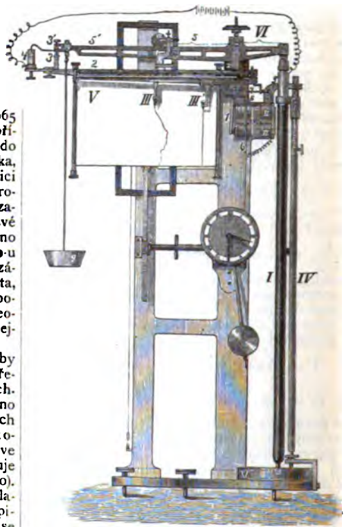
Č. 456. Barograf Sprungův.
